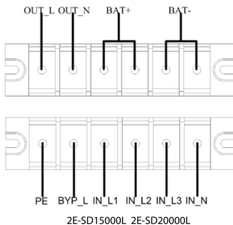
Мал. 2-1 Схема підключення клемного блоку
