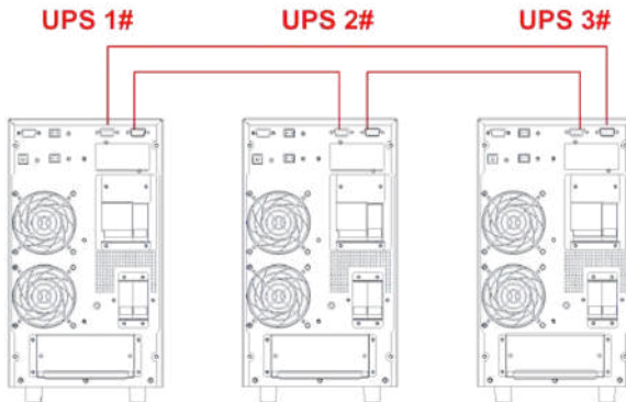
Мал. 2-4: Паралельна система 3 ДБЖ
