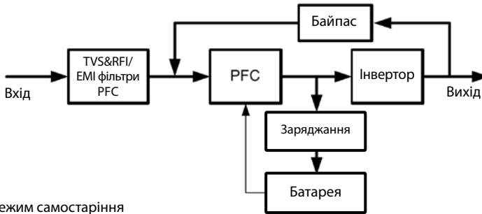
Мал. 1-8. Режим самостаріння
