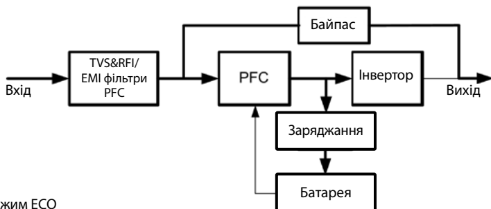
Мал. 1- 7: Режим ECO
