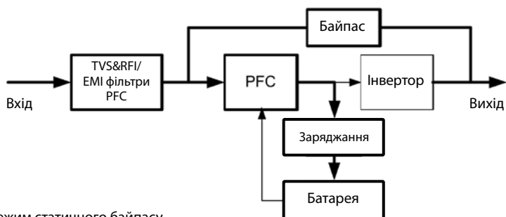
Мал. 1- 5: Режим статичного байпасу
