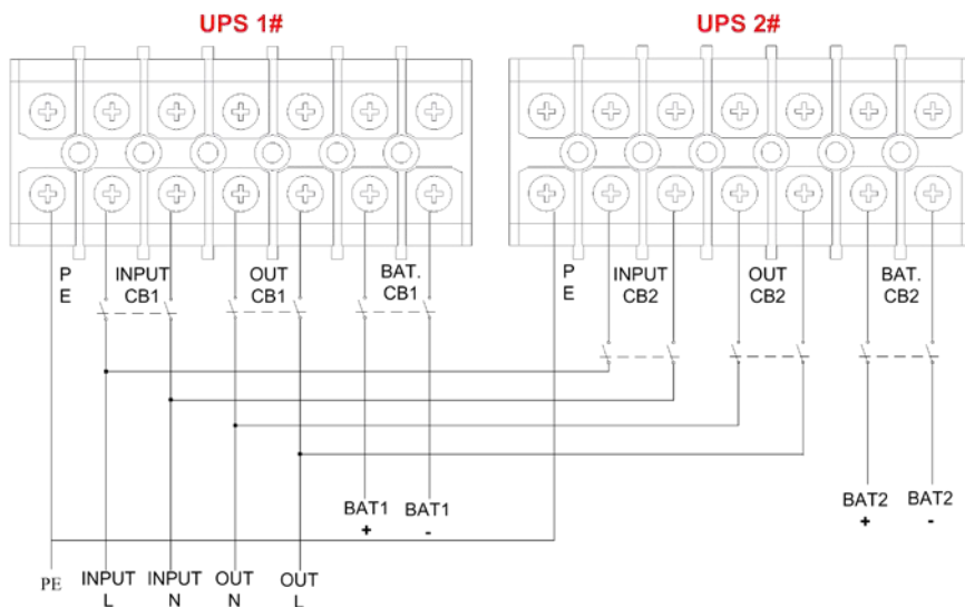
Мал. 2-2: Схема паралельного підключення
