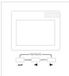
Мал. 3-1: Панель дисплея
