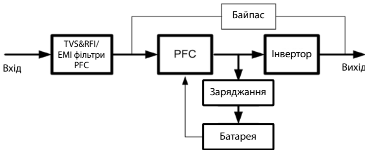
Мал. 1- 4: Нормальний режим
