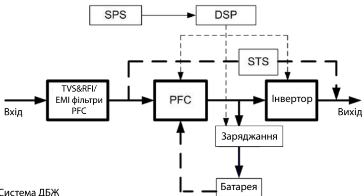
Мал. 1- 3: Система ДБЖ
