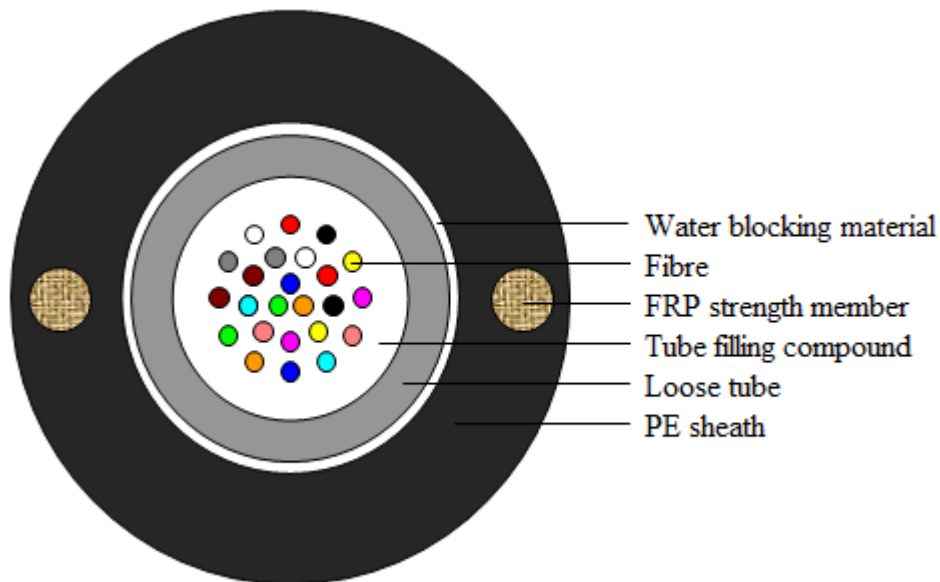
GYFXTY-24B1.3
